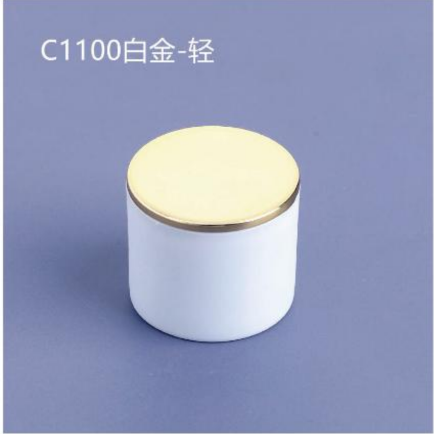
型号： 1100白金-轻 口径： 15mm/φ17.2 尺寸： 31*27
