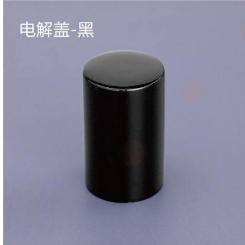
型号： 电解盖-黑 口径： 15mm/φ17.2 尺寸： 20*32
