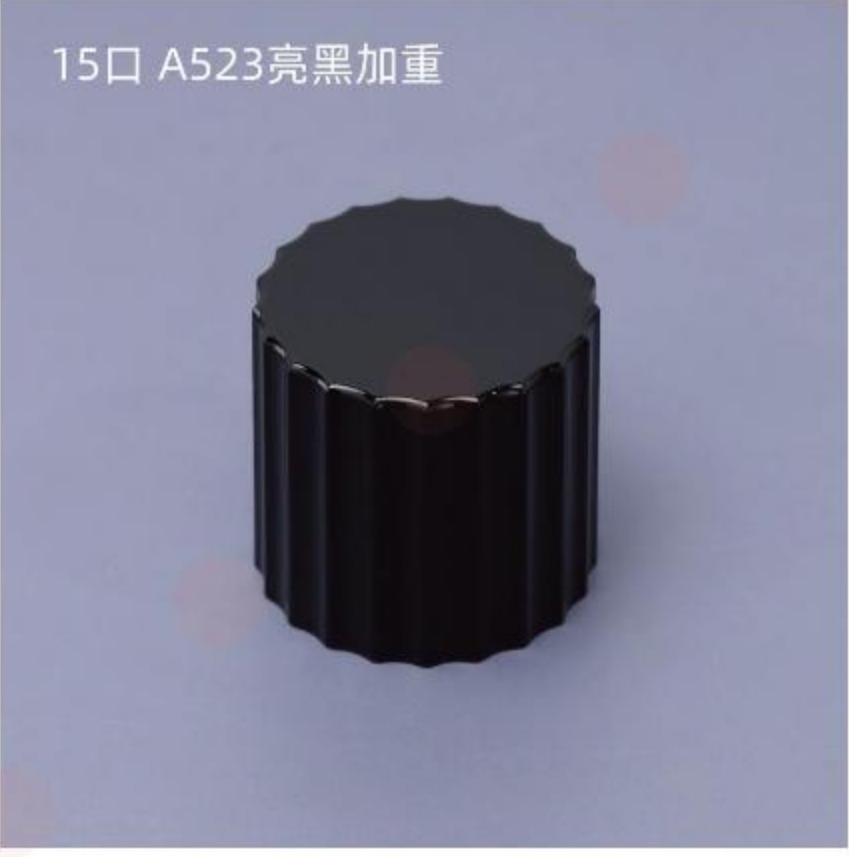
型号： A523亮黑加重 口径： 15mm/φ17.2 尺寸： 31*30
