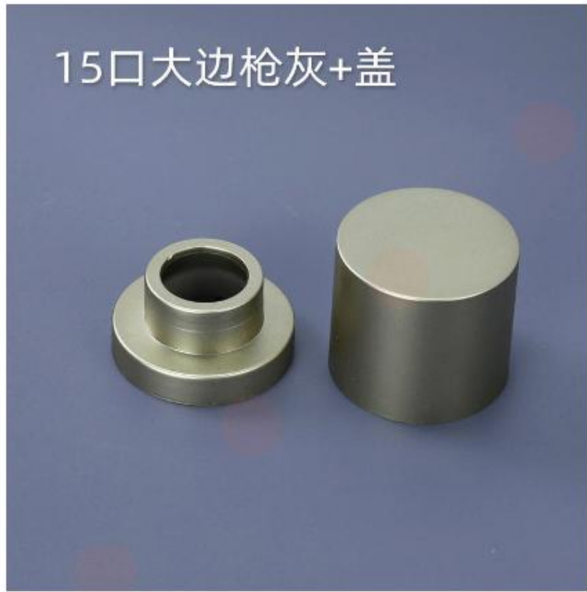
型号： 枪灰色盖 口径： 15mm/φ17.2 尺寸： 30*32
