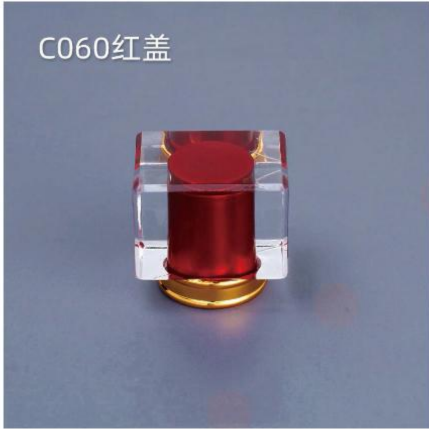
型号: C060红 口径: 15mm/φ17.2 尺寸: 36*29*35
