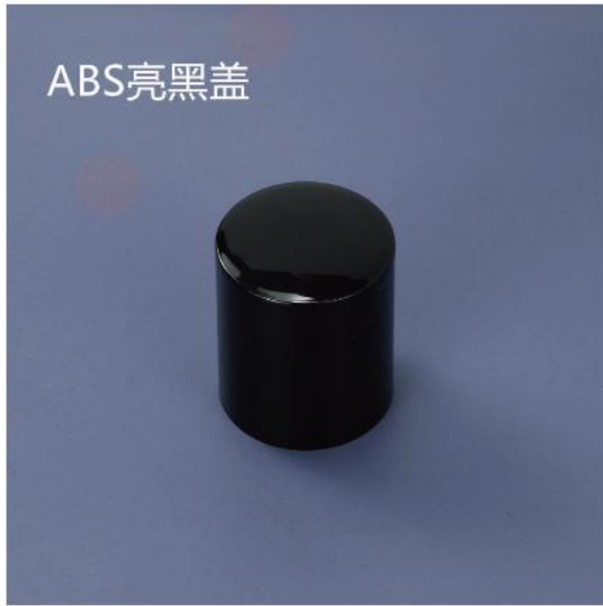
型号: 238亮黑盖-加重 口径: 15mm/φ17.2 尺寸: 25*29
