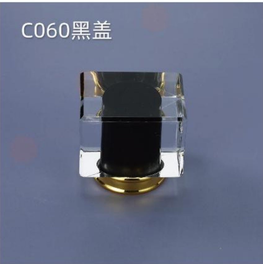
型号: C060黑 口径: 15mm/φ17.2 尺寸: 36*29*35
