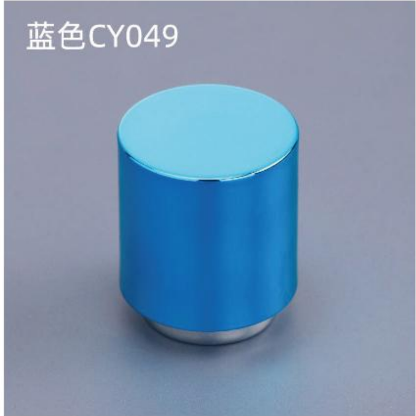
型号: CY049 口径: 15mm/φ17.2 尺寸: 27*32
