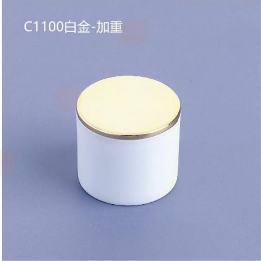
型号： 1100白金加重 口径： 15mm/φ17.2 尺寸： 31*27
