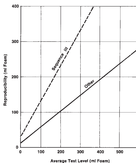
FIG. 4 Precision Chart—Reproducibility
