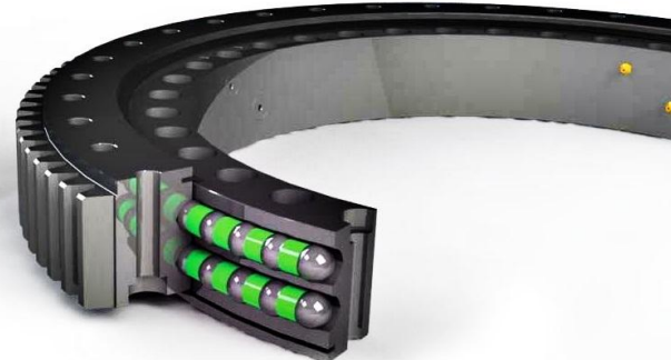
无齿式八点接触球转盘轴承
