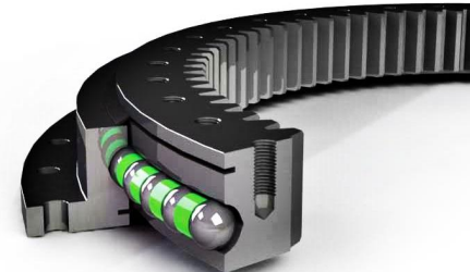
内齿式四点接触球转盘轴承
