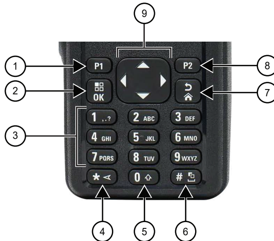
Gambar 7: Gambaran Umum Keypad
