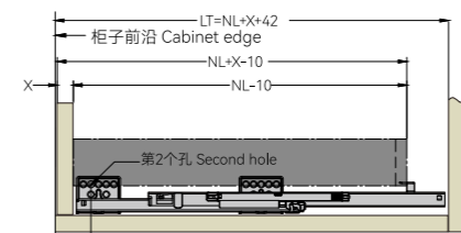
内置抽屉 Internal drawer
