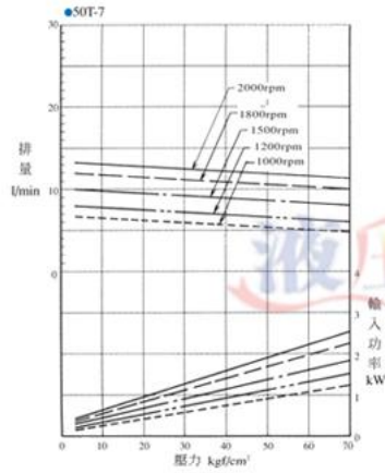
压力-排量·输入功率特性 作动油黏度20cSt
