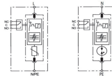
L-N/PE (1P)
