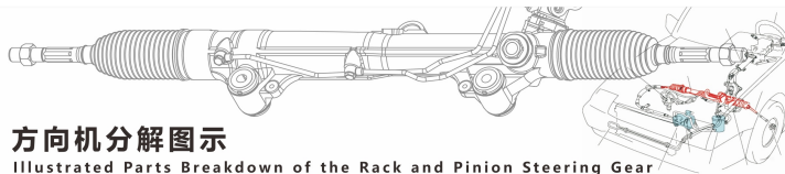
高尔夫电动车转向器 Golf Electric Steering Rack
