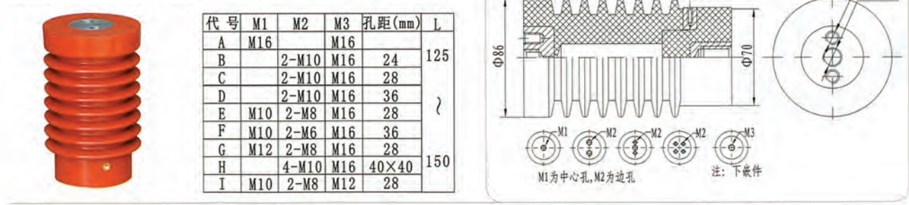
名称: 12kV 传感器 型号: CG12-01
