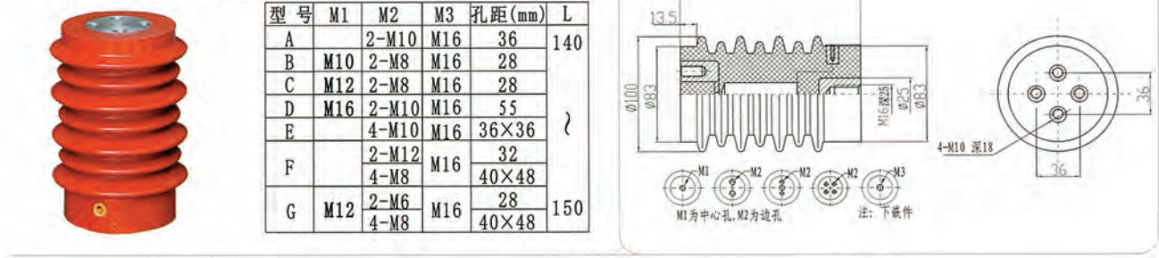
名称: 12kV 传感器 型号: CG12-03
