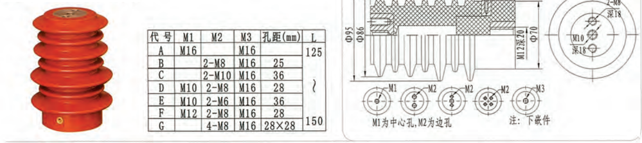
名称: 12kV 传感器 型号: CG12-02
