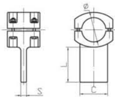
管母线T型线夹 (MGT(D)型)
