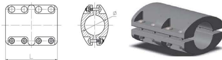
管母线外接头 (MJ (W) 型)
