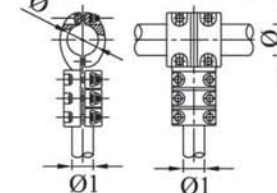
管母线T型线夹 (MGTL型)
