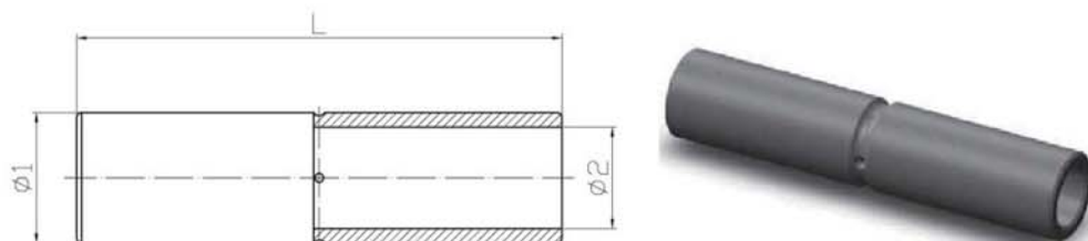
管母线内接头 (MJ 型)
