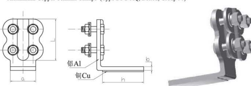
铜铝过渡设备线夹 (90° SLG-CQ螺栓型)
