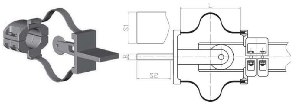
支撑式双伸缩设备线夹 (MSY型)
