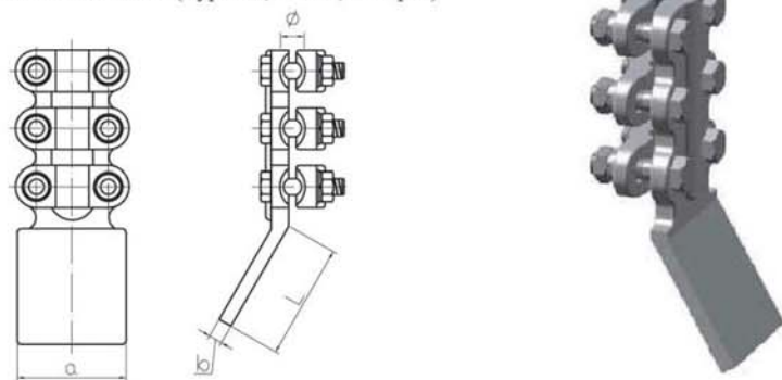
螺栓型设备线夹 (SL型B类)
