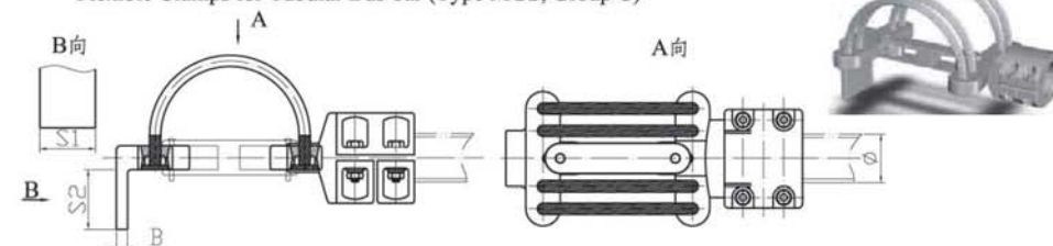
管母线伸缩线夹 (MGS型C类)
