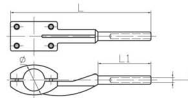
管母线T型线夹 (MGTY型)
