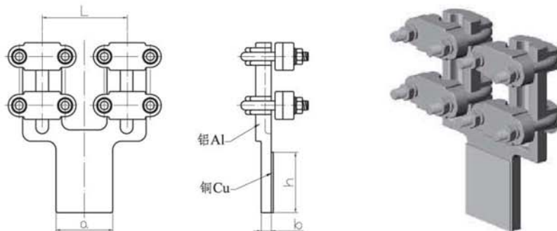
铜铝过渡双导线设备线夹 (0° 覆铜搪锡 SLSG 螺栓型)
