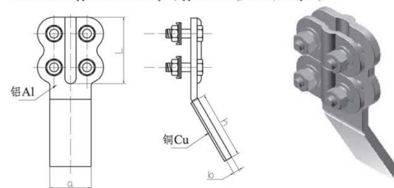
铜铝过渡设备线夹 (30° SLG-BQ螺栓型)
