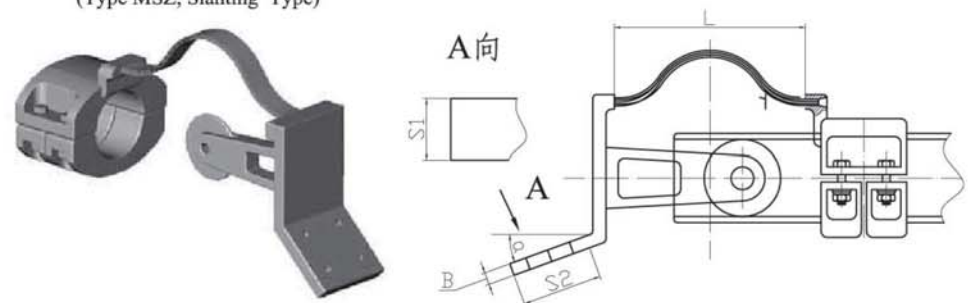
支撑式管母线单伸缩设备线夹 (MSZ型斜放式)
