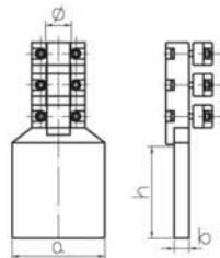
大截面导线设备线夹 (0° SL螺栓型) Terminal Clamps (Type SL)
