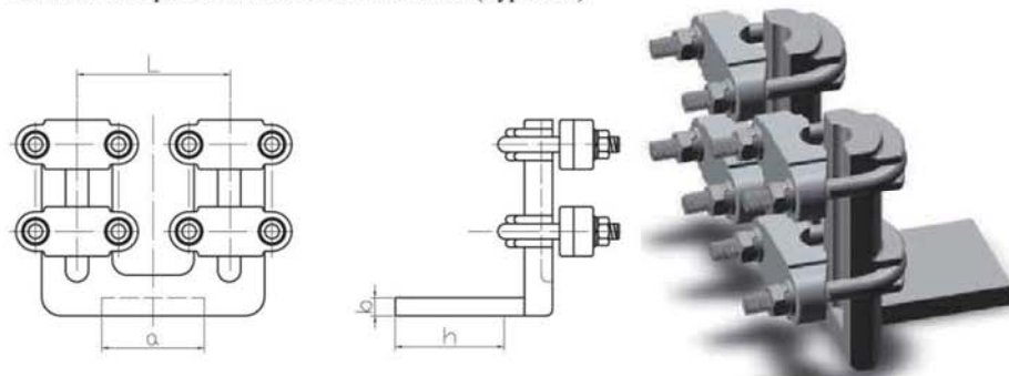
双导线设备线夹 (90° SLS 螺栓型)
