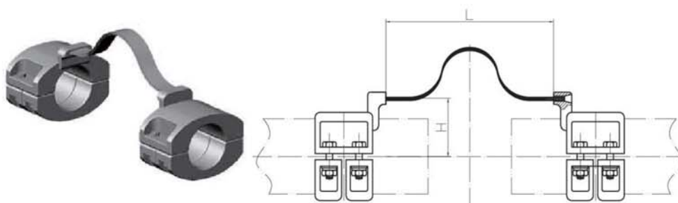
单伸缩引流线夹 (MGS 1 型)
