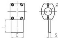
管母线T型线夹 (MGT型)
