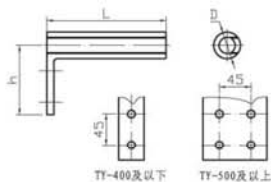
T型线夹 (TY/TY2液压型)
