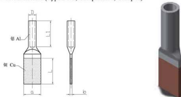
铜铝过渡设备线夹 (SYG压缩型A类)
