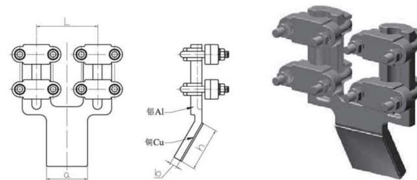
铜铝过渡双导线设备线夹 (30° 覆铜搪锡 SLSG 螺栓型)
