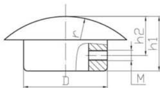
管母线封端盖 (MGF型)
