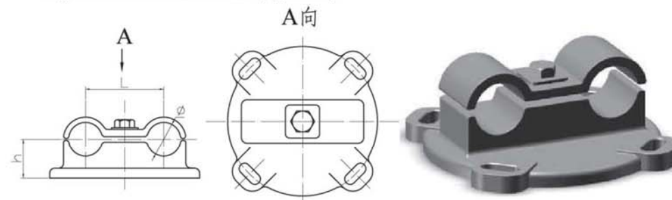
软母线固定金具 (MDG型双母线用)
