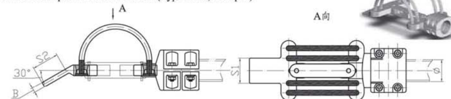
管母线伸缩线夹 (MGS型B类)
