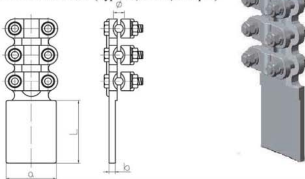
螺栓型设备线夹 (SL型A类)
