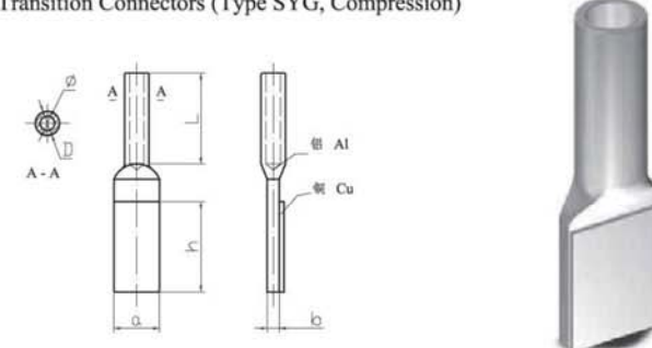
铜铝过渡设备线夹 (A覆铜搪锡)
