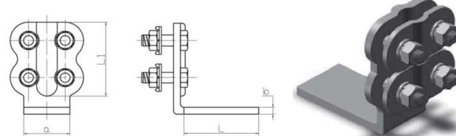
螺栓型设备线夹 (SL型C类)
