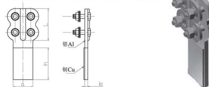
铜铝过渡设备线夹 (0° 覆铜搪锡, SLG-AQ螺栓型)
