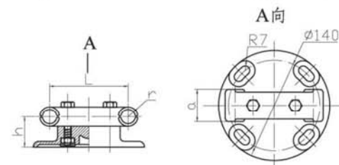
软母线固定金具 (MDG型双母线用)
