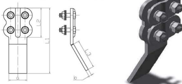
螺栓型设备线夹 (SL型B类)
