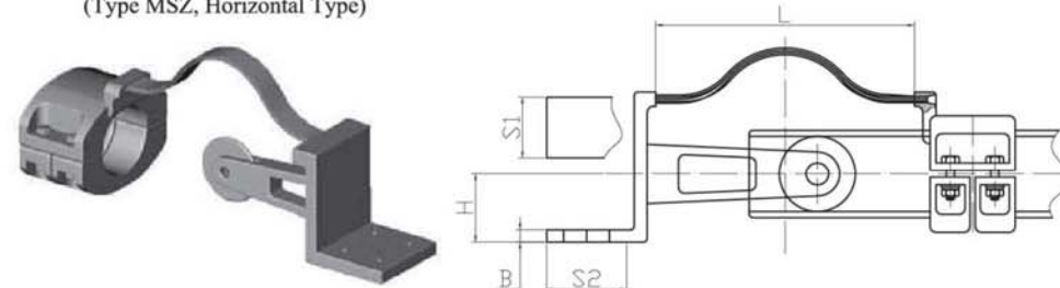
支撑式管母线单伸缩设备线夹 (MSZ型平放式)
