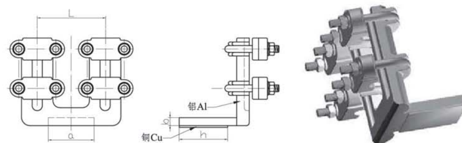
铜铝过渡双导线设备线夹 (90° 覆铜搪锡 SLSG 螺栓型)
