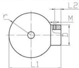
管母线封端球 (MGZ型)
