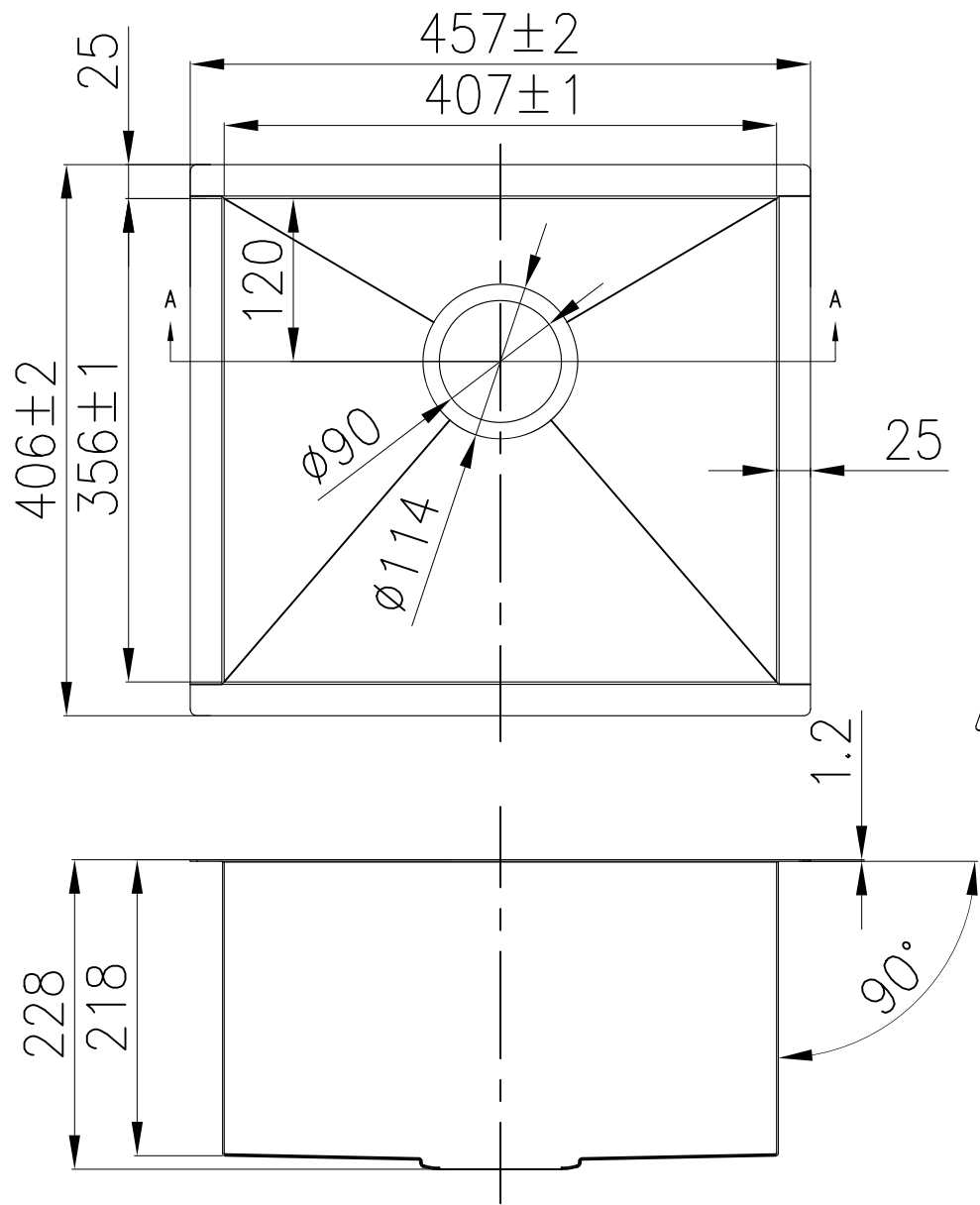
剖面 A-A
