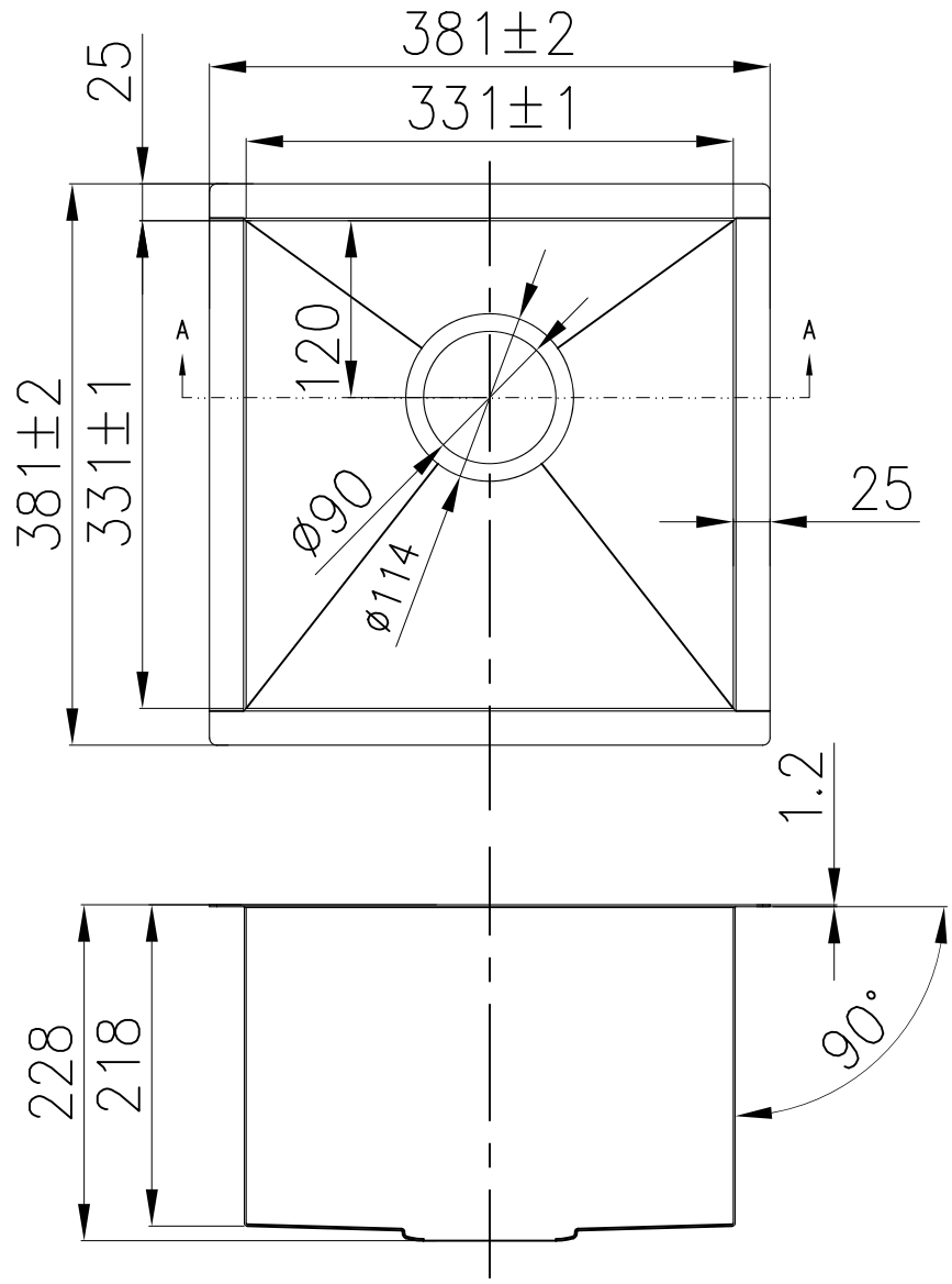
剖面 A-A
