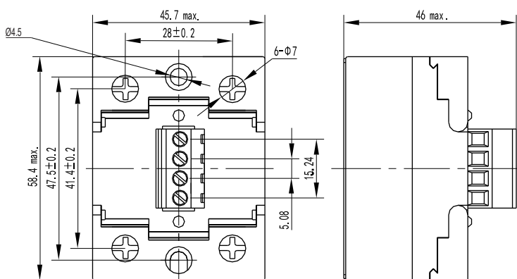
Bolt terminal(IP20)
