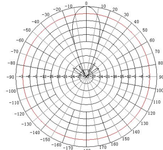
H-Plane
