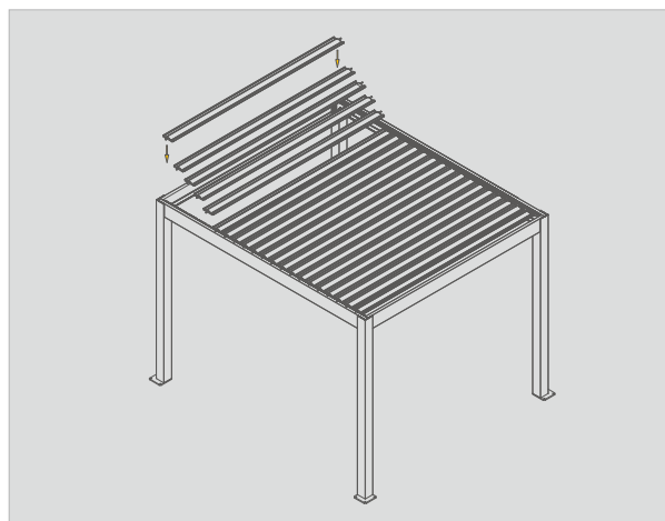
03 安装叶片
