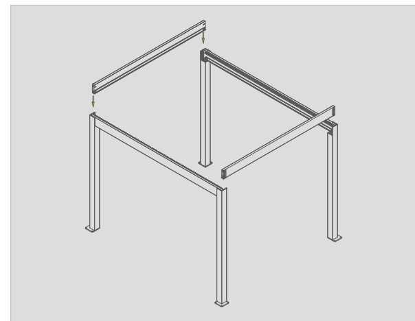
02 拼接边框
