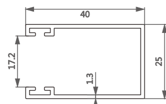
型号/Item No.-0901586 米重/Weight-0.424kg/m
