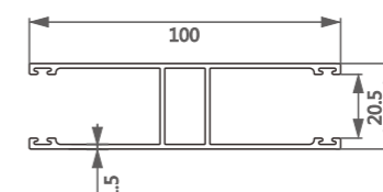
型号/Item No.-79081016-1.5 米重/Weight-1.116kg/m
