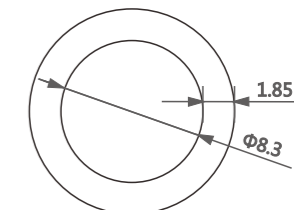
型号/Item No.-6110446 米重/Weight-0.16kg/m
