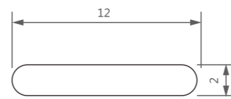
型号/Item No.-920010 米重/Weight-0.063kg/m
