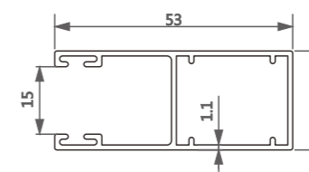
型号/Item No.-4278082 米重/Weight-0.515kg/m
