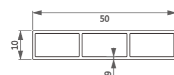
型号/Item No.-4237164 米重/Weight-0.331kg/m
