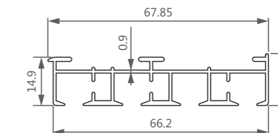
型号/Item No.-1514180 米重/Weight-0.548kg/m
