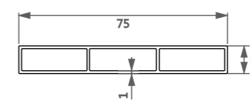
型号/Item No.-4237165 米重/Weight-0.497kg/m
