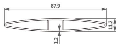
型号/Item No.-7908359 米重/Weight-0.621kg/m
