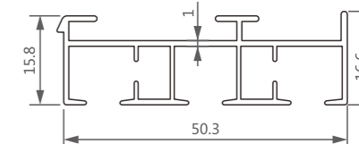
型号/Item No.-1514180 米重/Weight-0.548kg/m
