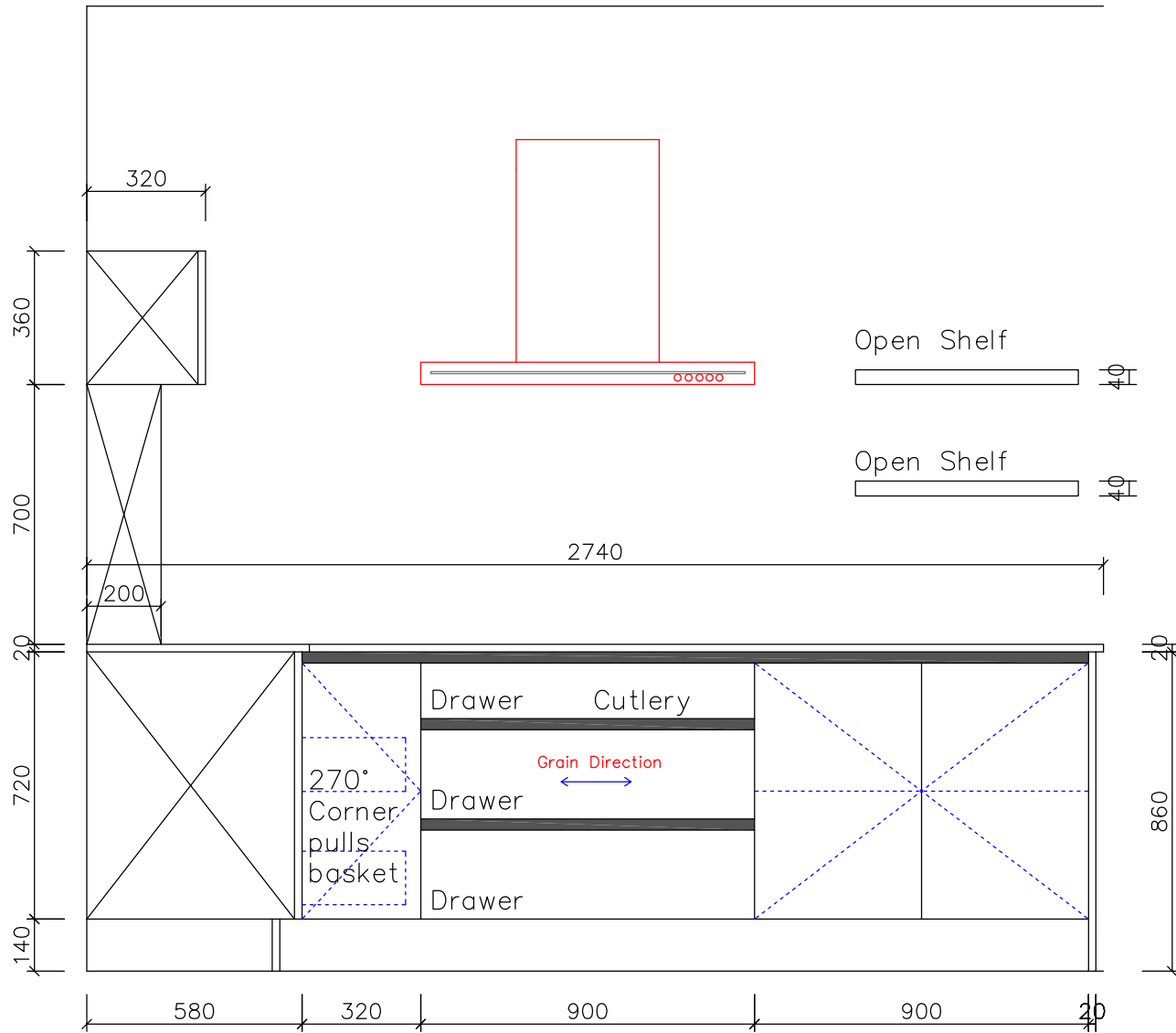
Elevation B
