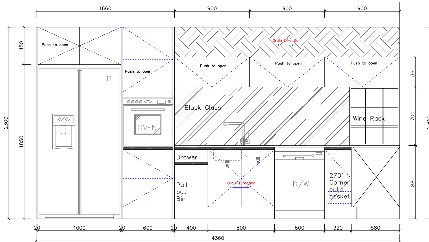
Elevation A
