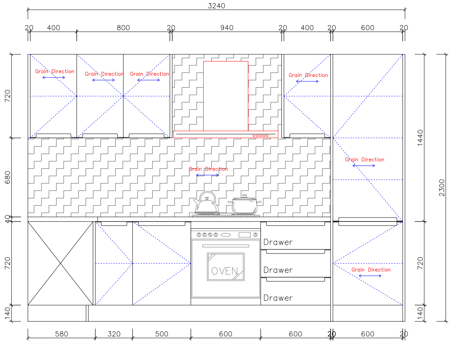
Elevation B
