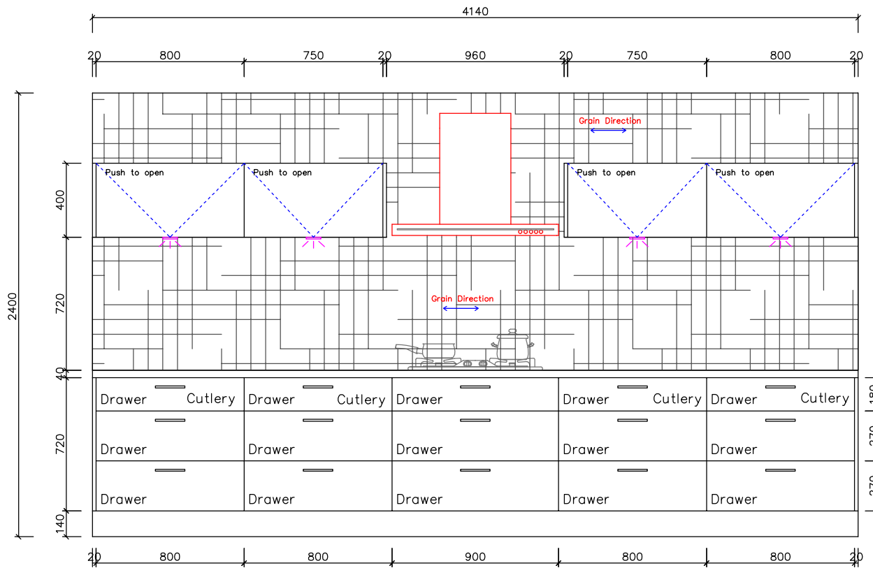
Elevation A
