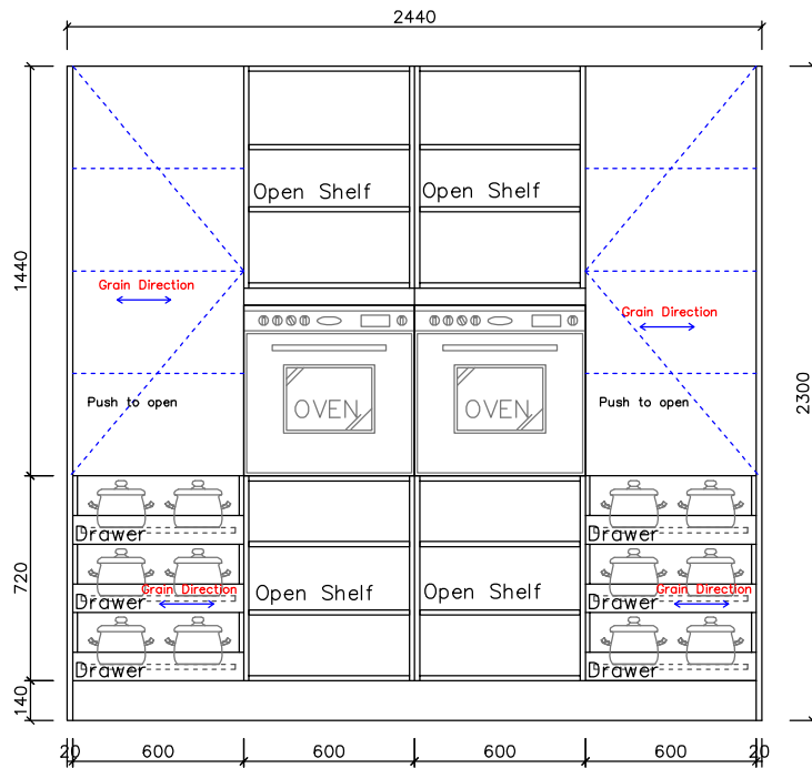
Elevation B
