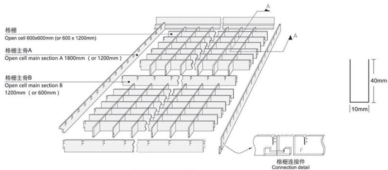
格栅天花安装示意图 Combination open cell ceiling installation diagram
