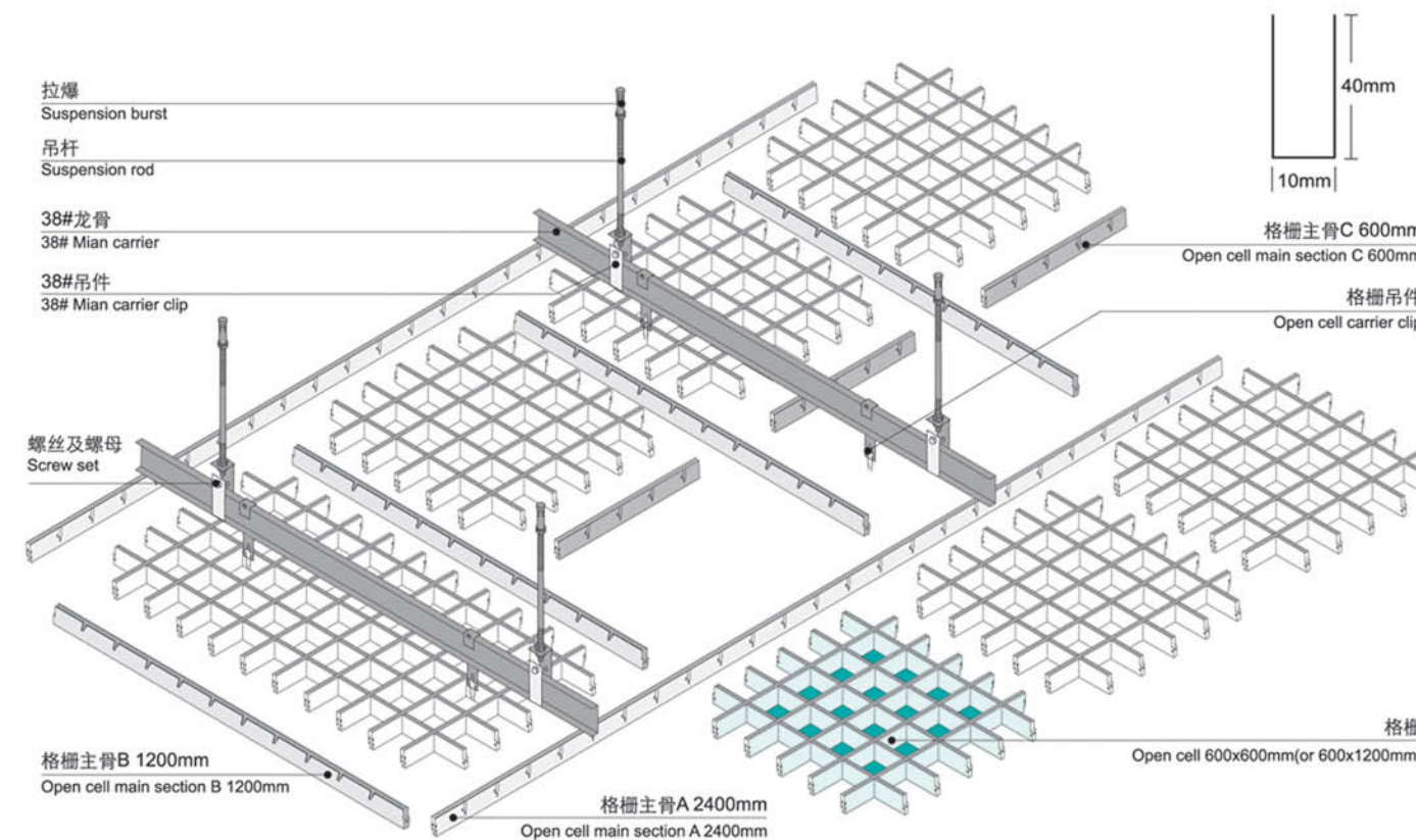
格栅天花安装示意图 Combination open cell ceiling installation diagram
