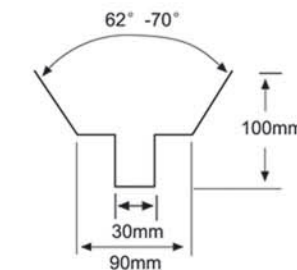
超高身异型格栅侧面示意图 Super high pyramid open cell ceiling
