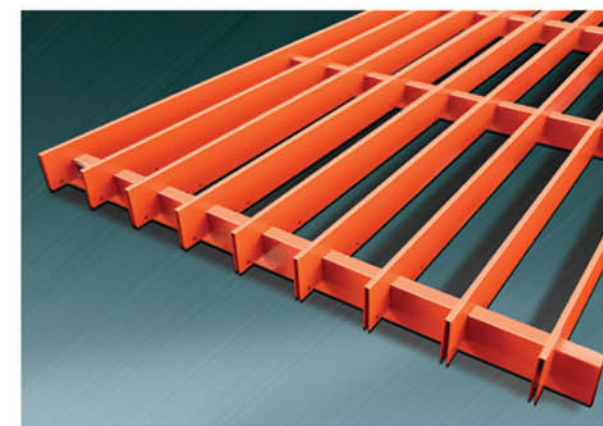
■ 高低镀锌铁组合格栅 Galvanized iron combination open cell 主骨Main section : 宽度Width 4.5mm , 高度Height 43mm , 长度Length 1250mm 副骨Cross section : 宽度Width 14.5mm , 高度Height 38mm , 长度Length 600mm
