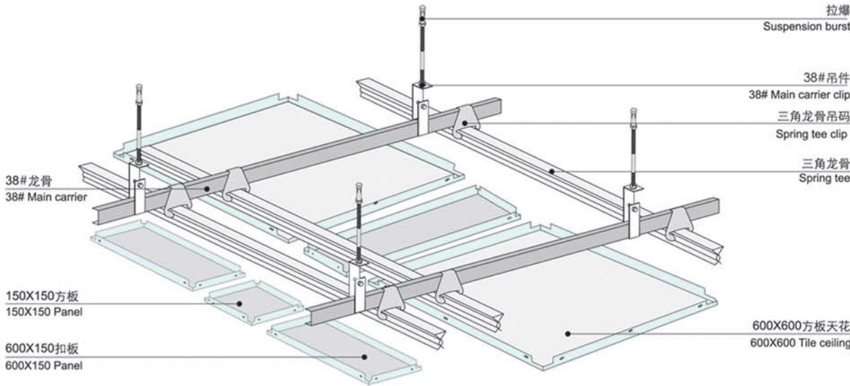
普通组合板天花安装图 Combination ceiling installation diagram
