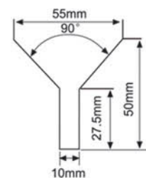
异型高身格栅侧面示意图 High pyramid open cell ceiling
