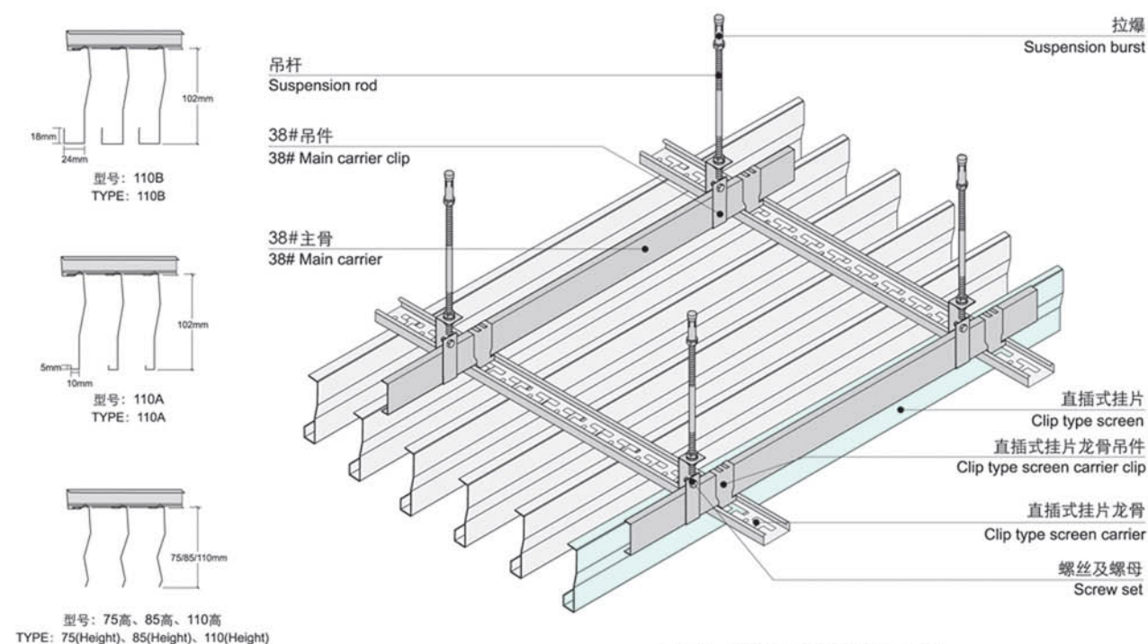
直插入式挂片天花安装示意图 Clip type screen ceiling installation diagram
