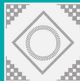
TDL-25 \phi 2.5孔拼花 TDL-25 \phi 2.5 match punching
