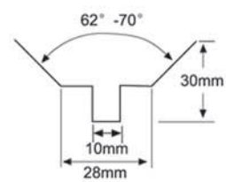
异型矮身格栅侧面示意图 Low pyramid open cell ceiling
